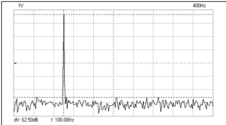
DHT à 100 Hz :
