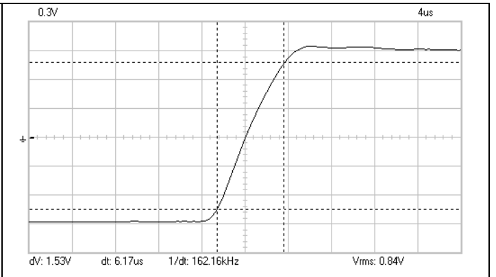
Temps de montée : 6,2 \mu Sec
