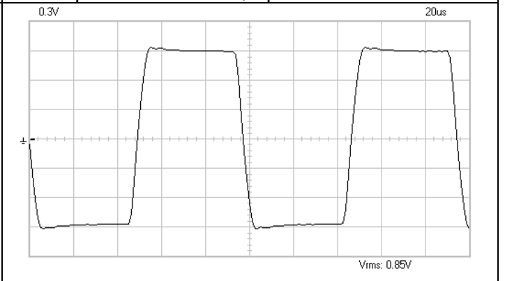
Carré à 10 KHz
