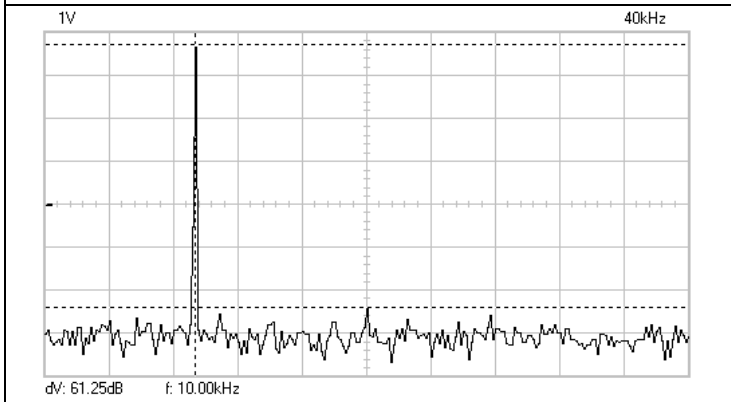
DHT à 10 KHz
