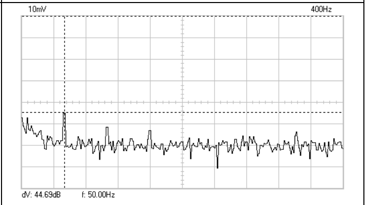
Hum 50 & 100 Hz : -84 dBV (44 db / 10 mV)
